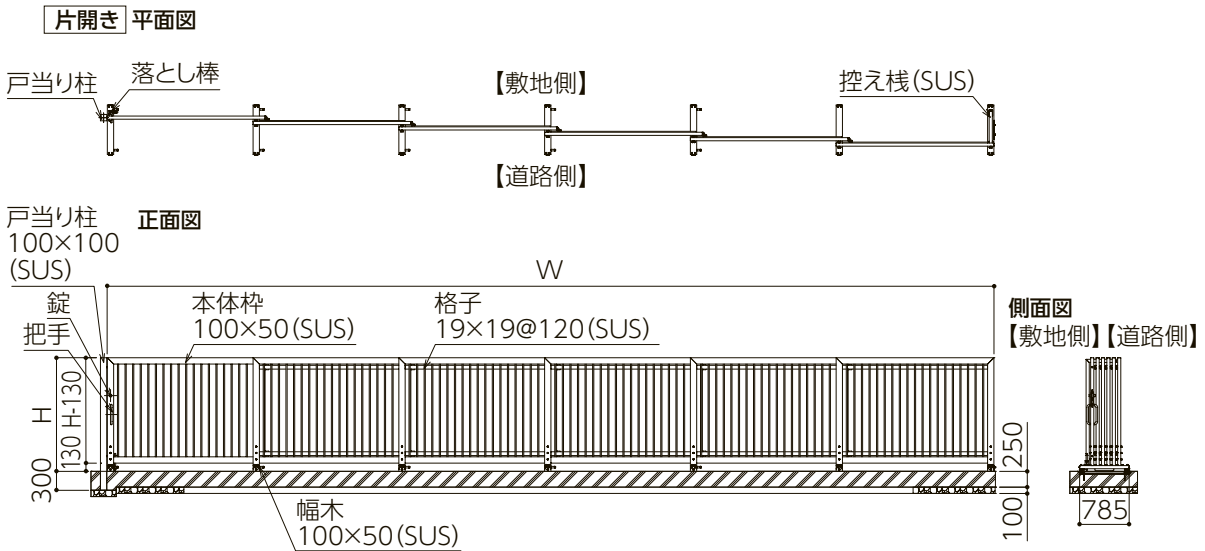
■複連引戸S型(片開き) サイズ表
