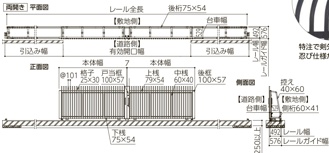
■A2型 ステンレスフラットレールタイプ〈片開き〉サイズ表
