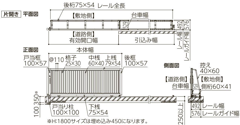
■A1型 ステンレスフラットレールタイプ(片開き) サイズ表
