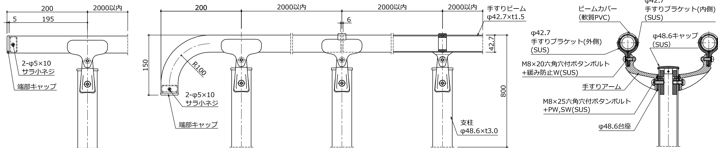
組付詳細図 S=1:4
