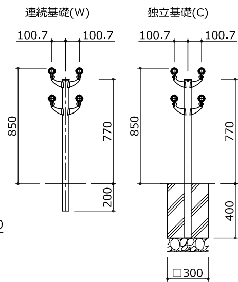
側面図 S=1:20
